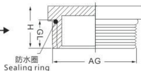
电缆接头 分解示意图 Cable connector Decomposition diagram
