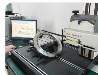
Mahr Profilometer
